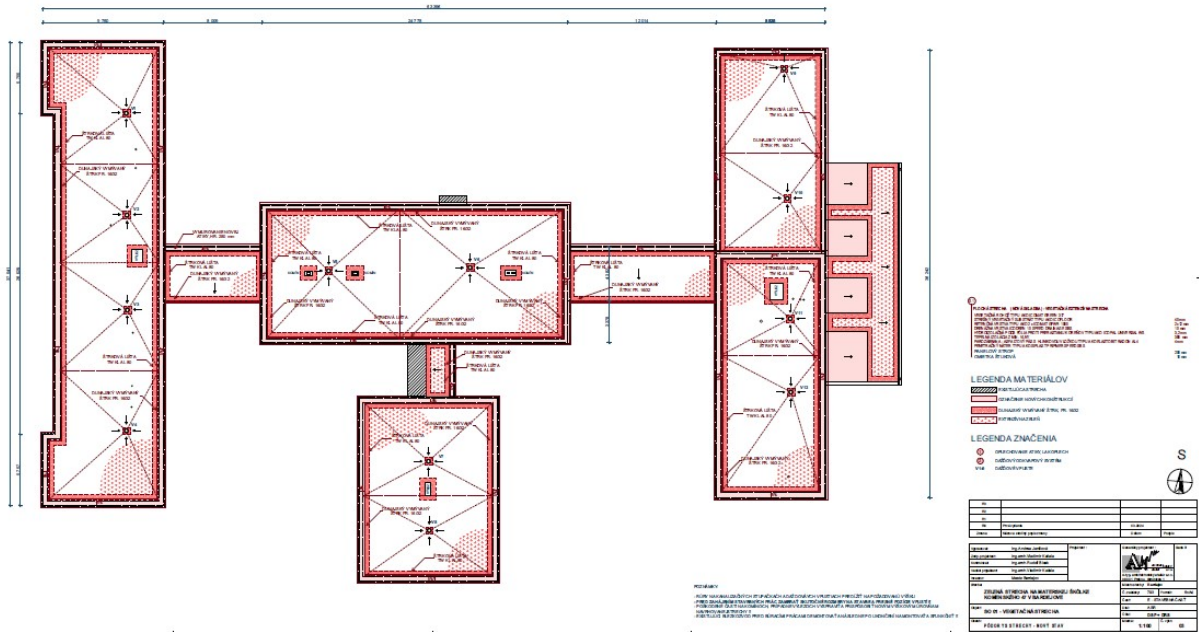
Obr.1: Zelená strecha na Materskej škôlke Nábrežná 2 v Bardejove
