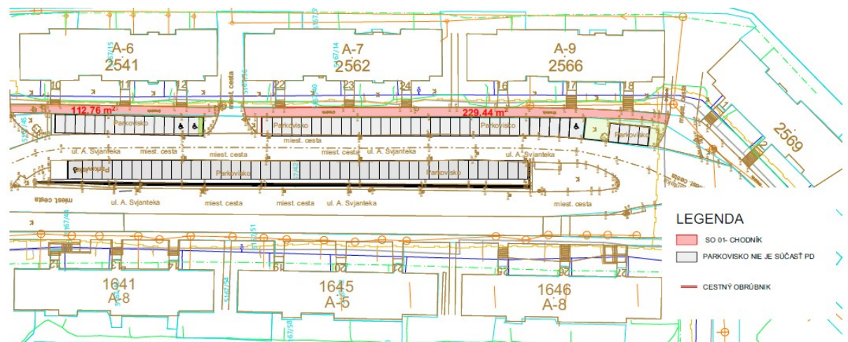
Obr.6: Zelené parkovisko sídlisko Vinbarg - ul. A. Svianteka 10, 11, 15, 22-24, 16-18 v Bardejove- chodníky
