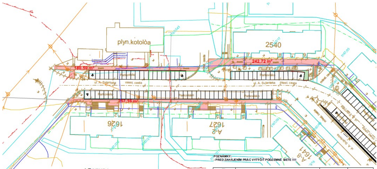
Obr.4: Zelené parkovisko sídlisko Vinbarg - ul. A. Svianteka 1 - 9 v Bardejove - chodníky
