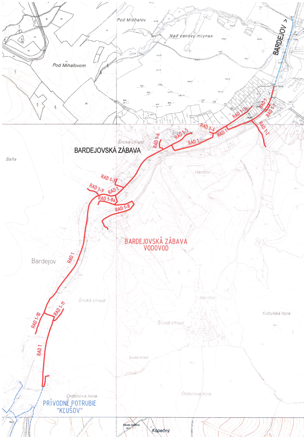
Obr. Celková situácia stavby
